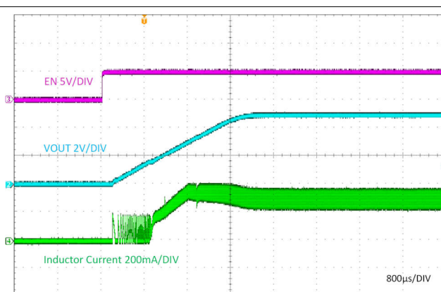
図 8-6. Start-Up by EN
