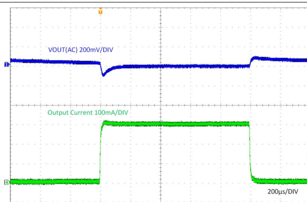
図 8-8. Load Transient (0mA – 300mA)
