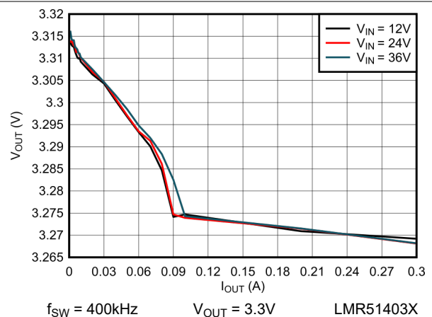
図 6-6. 3.3V Load Regulation
