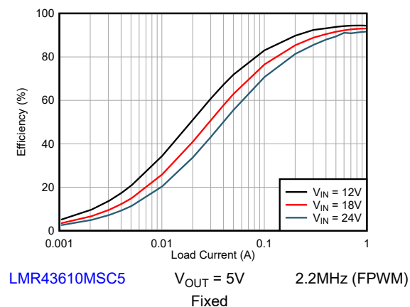
図 8-6. Efficiency
