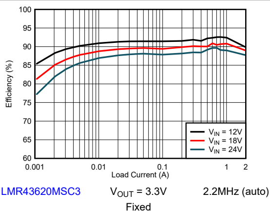
図 8-3. Efficiency
