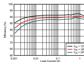
効率: V_{OUT} = 3.3V (固定)、2.2MHz
