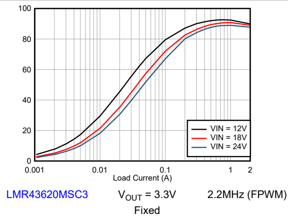
図 8-4. Efficiency
