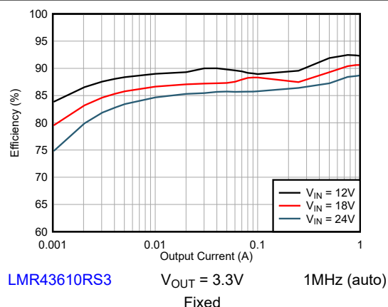
図 8-7. Efficiency
