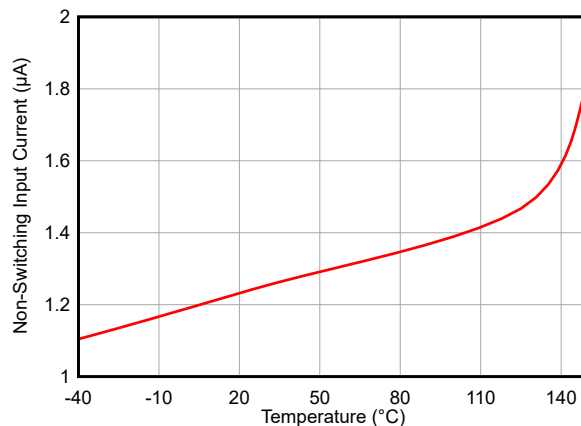
FIG 7-2. Nonswitching Input Current ( I_{qVIN(nonsw)} ) Versus Temperature
