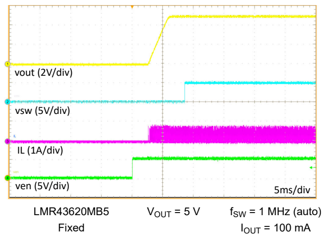
图 9-7. Start-up
