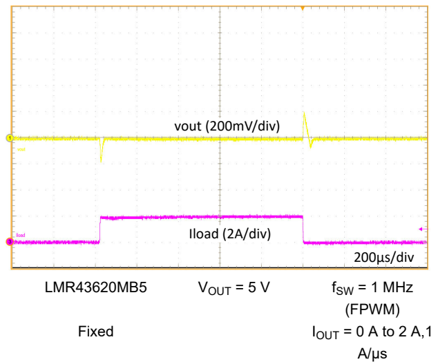
图 9-10. Load Transient
