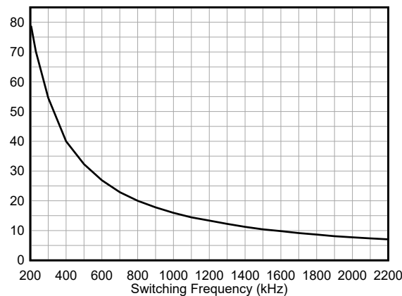
図 8-7. RT Values vs Frequency
