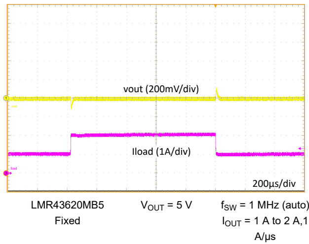
图 9-9. Load Transient
