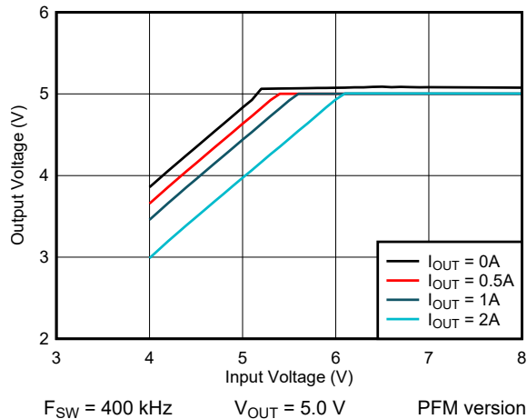
图 6-3. 5-V Dropout
