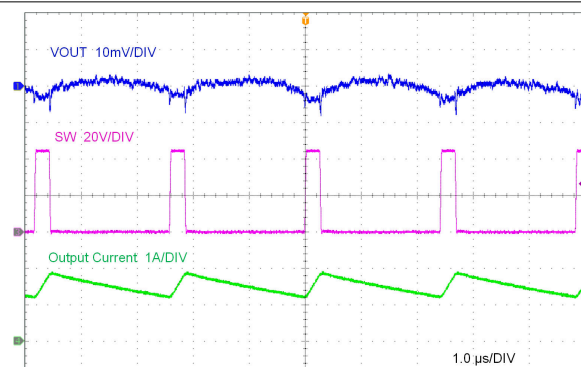
LMR38015-Q1 V_{OUT} = 5V AC 結合 400kHz
