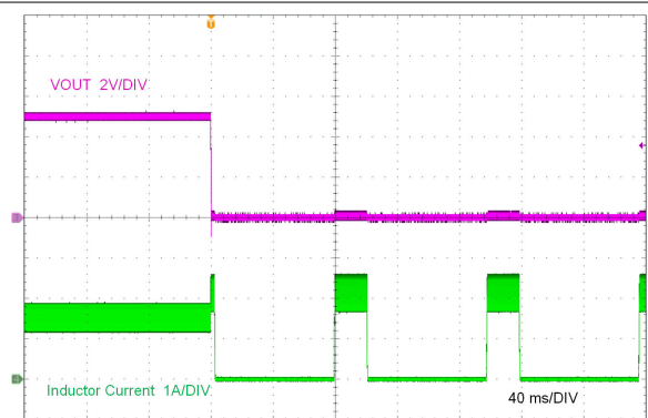
LMR38015-Q1 V_{OUT} = 5V 1 A から短絡
