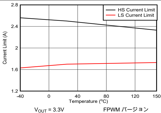
図 6-5. ハイスайдおよびローサイド電流制限と温度との関係
