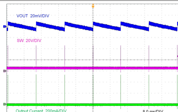
LMR38015-Q1 V_{OUT} = 5V AC 結合 無負荷
