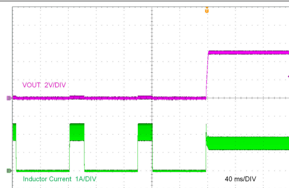
LMR38015-Q1 V_{OUT} = 5V 短絡から回復
