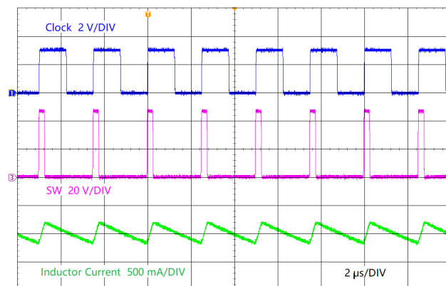
LMR38010-Q1 V_{OUT} = 5\text{ V} 400 kHz
