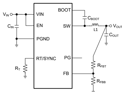
概略回路図
