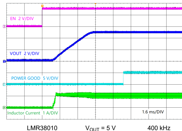
図 9-4. Start-Up by EN
