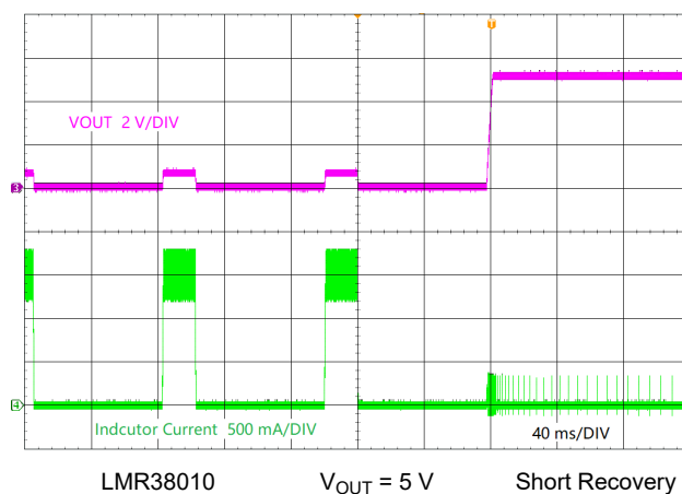
図 9-8. Short-Circuit Recovery
