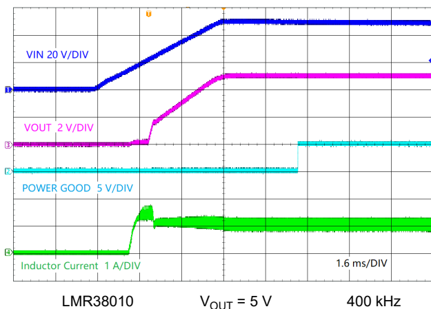
図 9-3. Start-Up by VIN
