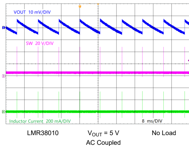
図 9-5. PFM Switching
