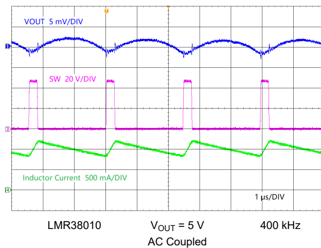
図 9-6. Full Load Switching
