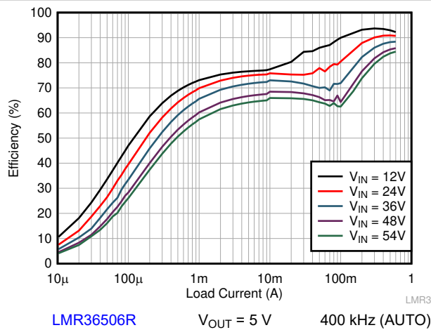
图 9-6. Efficiency
