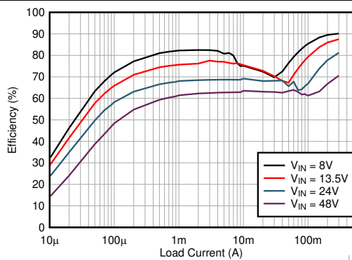
LMR36503MSC5 V_{OUT} = 5 V Fixed 2.2 MHz (AUTO)
