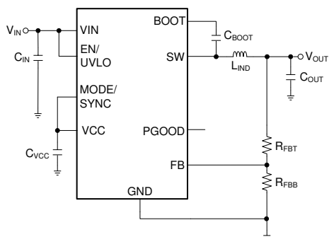
概略回路図
