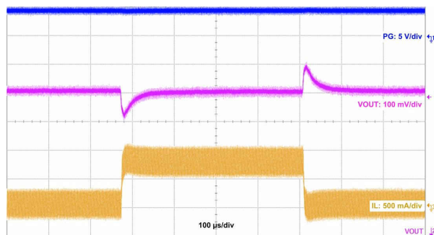
✎ 10-34. Load Transient
