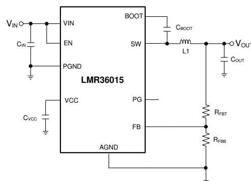
概略回路図
