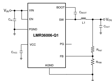
概略回路図
