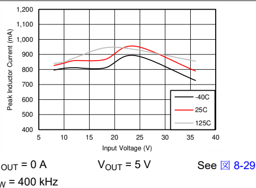
图 6-6. I PEAK-MIN
