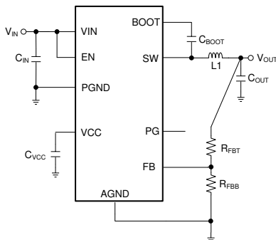
概略回路図
