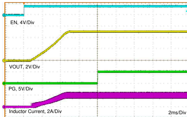
8-3. Precision Enable Behavior
