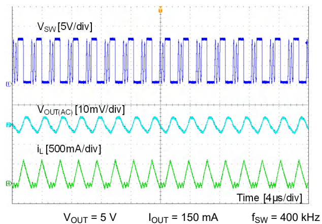
图 9-3. DCM Mode
