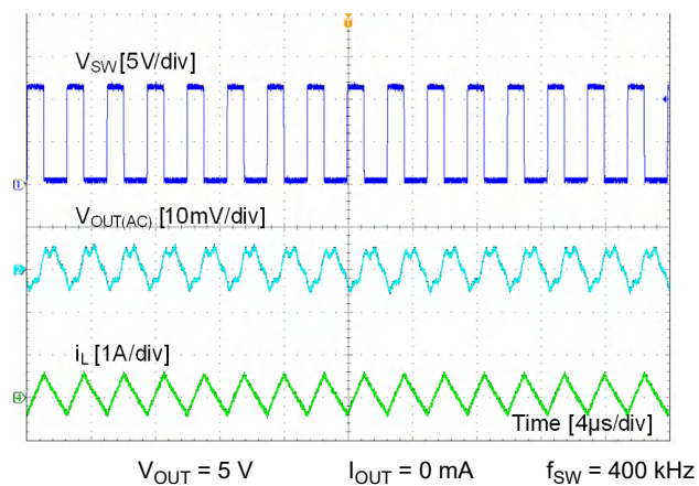
图 9-5. FPWM Mode
