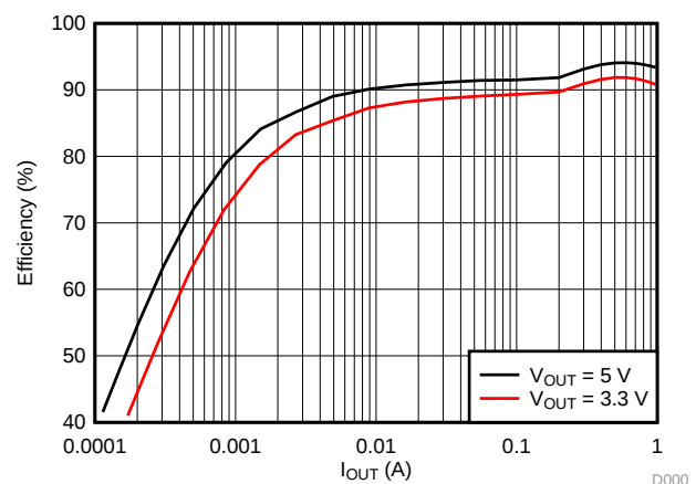
効率と負荷との関係、VIN = 12V
