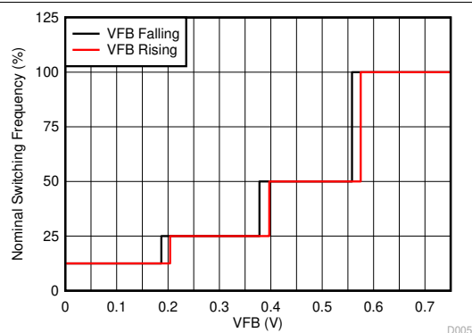
図 5-6. Frequency vs V_{FB}
