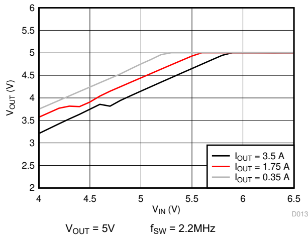
図 5-9. Dropout Curve
