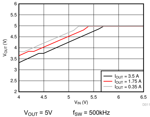
図 5-7. Dropout Curve
