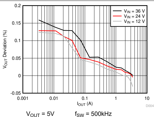
図 5-5. Load Regulation
