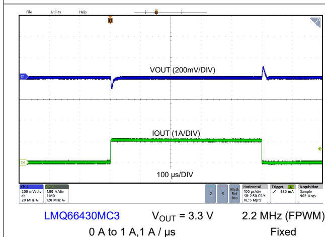
図 8-12. Load Transient
