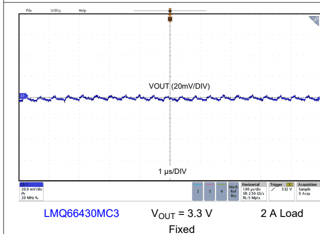
図 8-14. Output Voltage Ripple
