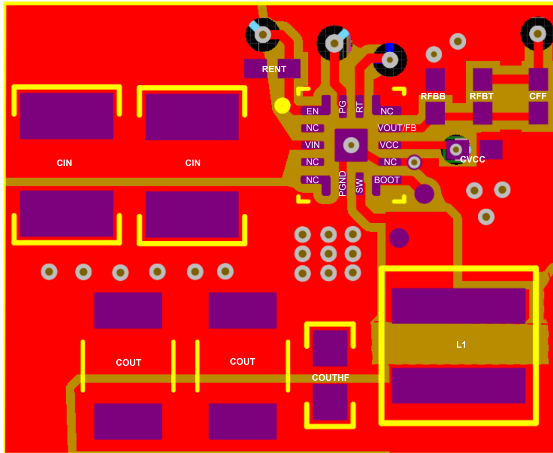
図 8-34. Example Layout
