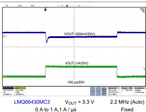
図 8-13. Load Transient
