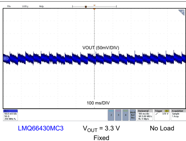
図 8-15. Output Voltage Ripple
