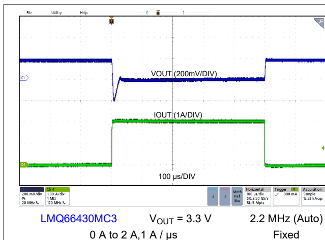
図 8-10. Load Transient
