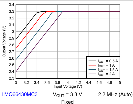
8-6. Dropout
