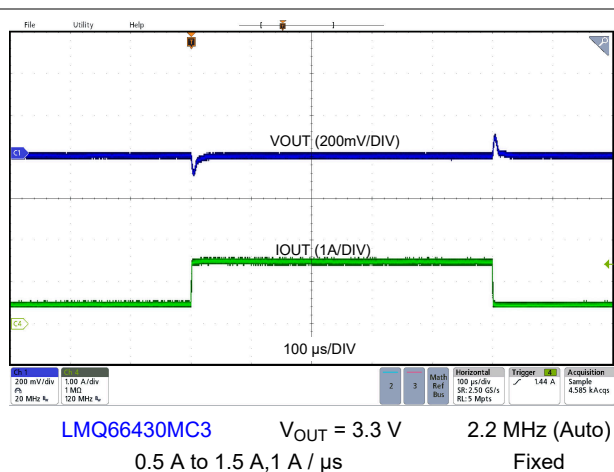
図 8-11. Load Transient
