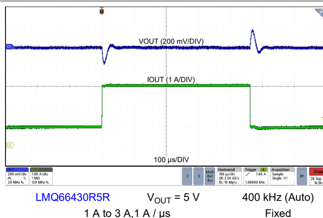
9-9. Load Transient
