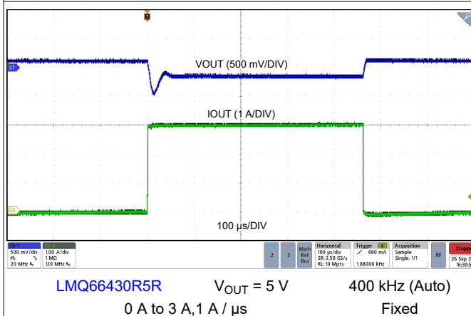
9-8. Load Transient
