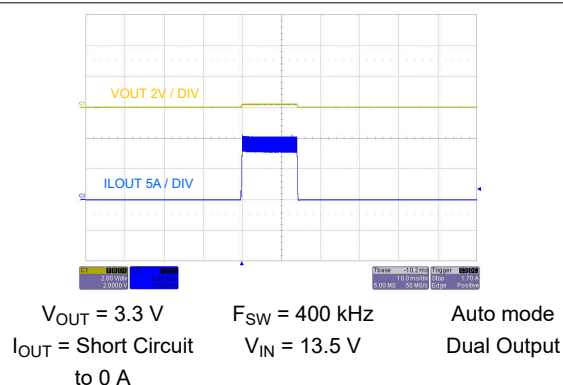
図 8-44. Short-Circuit Hiccup
