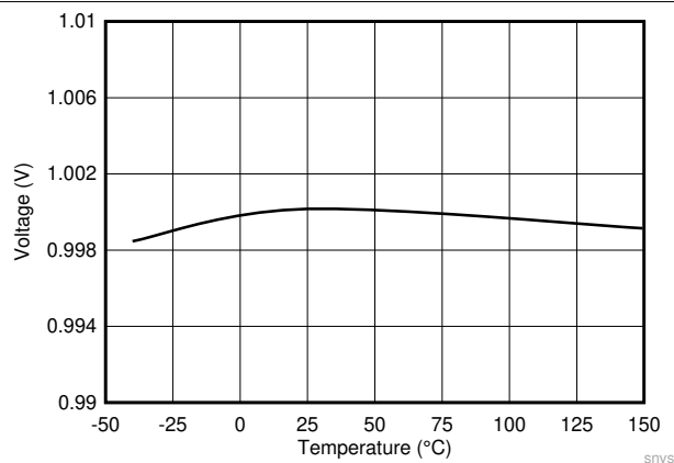
図 7-3. 帰還電圧
