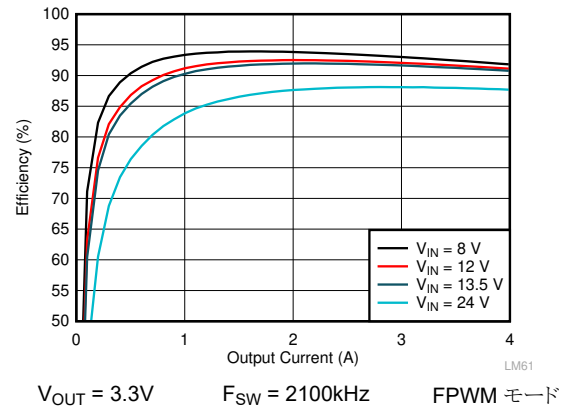
図 9-6. LMQ62440-Q1 の効率
