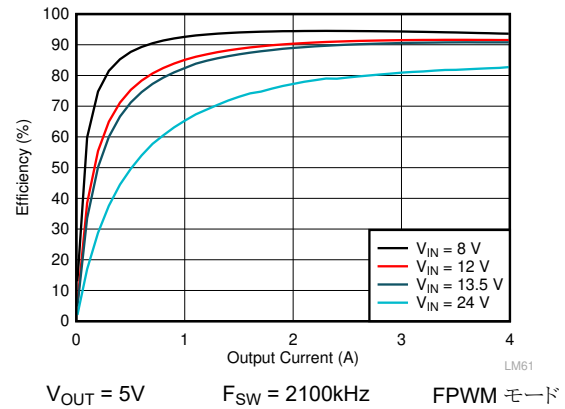
図 9-8. LMQ62440-Q1 の効率
