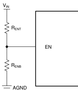
図 9-4. EN を使った UVLO
