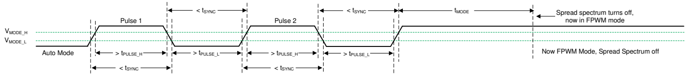
図 8-9. 自動モードから FPWM モードへの遷移でのスペクトラム拡散の無効化
