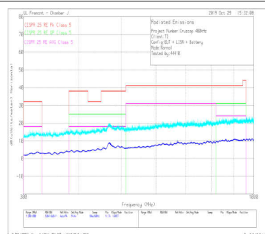
図 9-30. 放射 EMI (バイコニカル、水平) と CISPR25 制限値との関係
