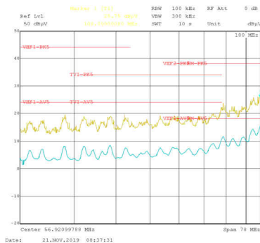
図 9-35. 伝導 EMI と CISPR25 制限値との関係 (黄 : ピーク信号、青 : 平均信号)
