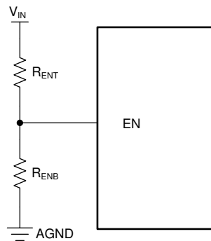
図 8-1. EN ピンを使った V_{IN} /UVLO
