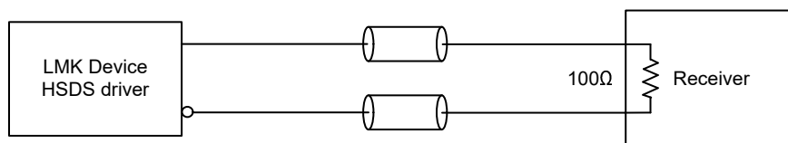
図 7-27. DC 結合 HSDS/LVDS 出力終端
