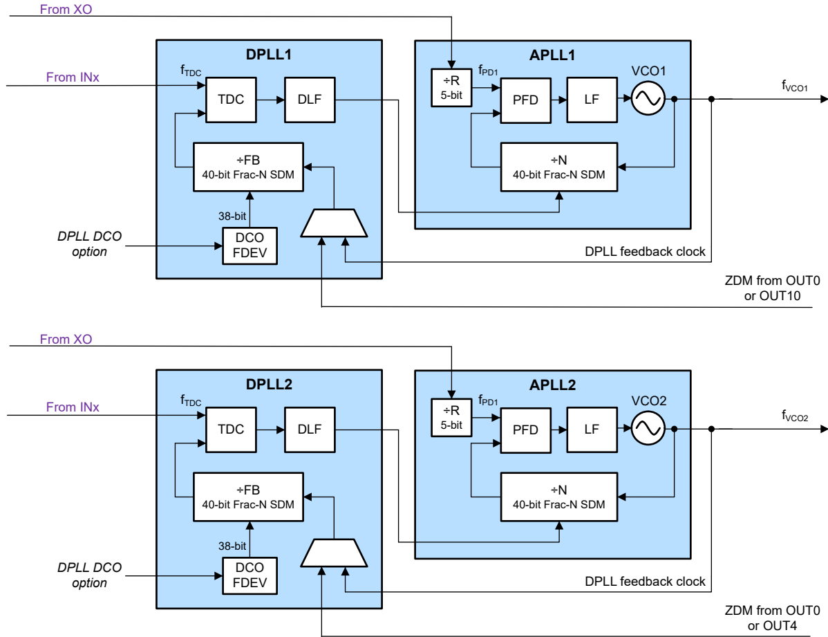
図 7-3. DPLL 動作
