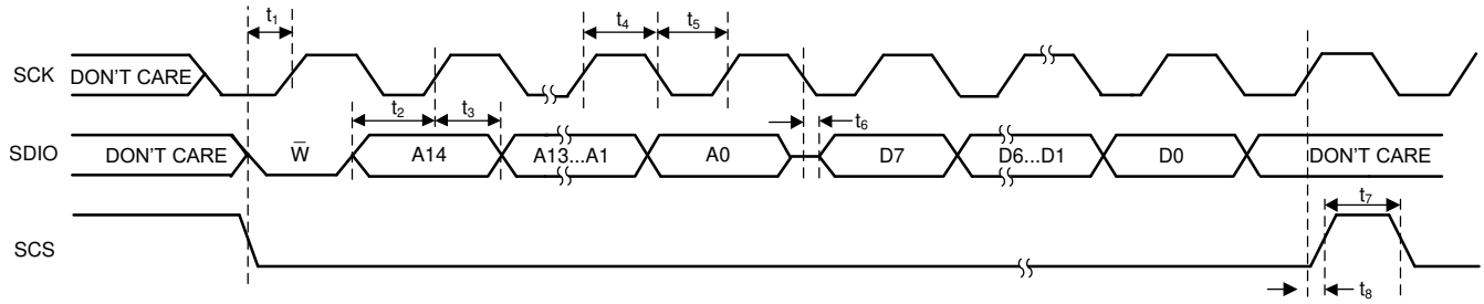
図 5-3. SPI 3 線式読み出しタイミング図
