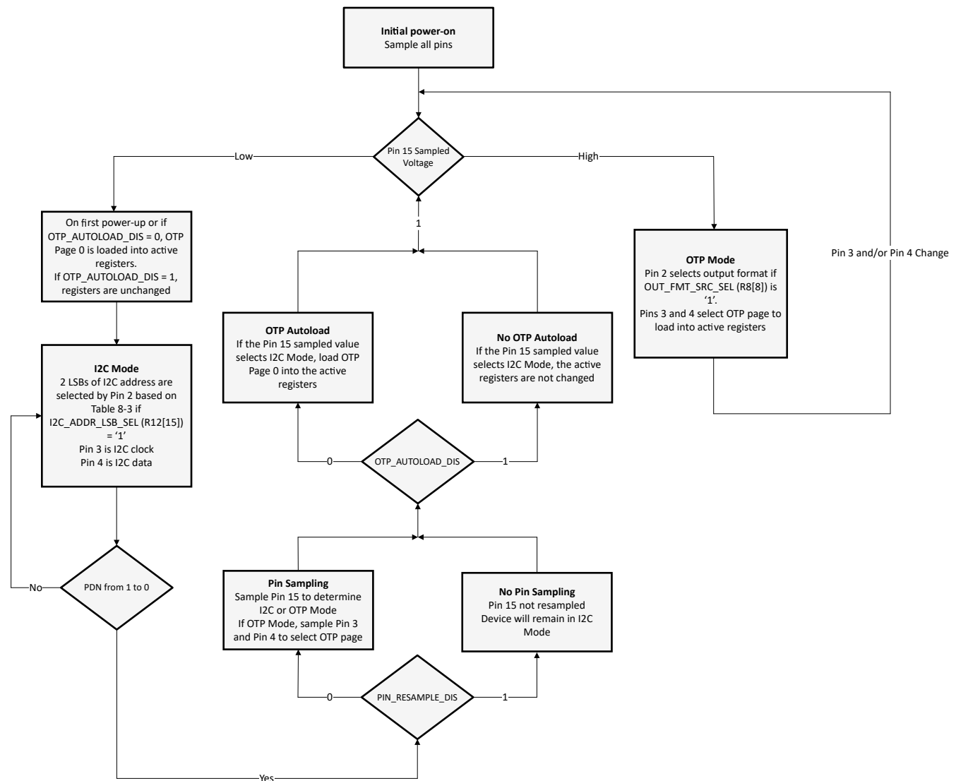
図 7-2. LMK3H0102 デバイスのモード図
