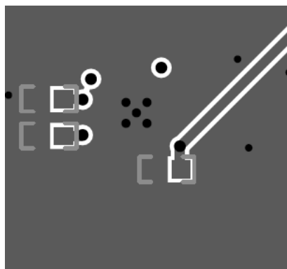
図 9-9. LMK3H0102 の PCB レイアウト例、最下層
