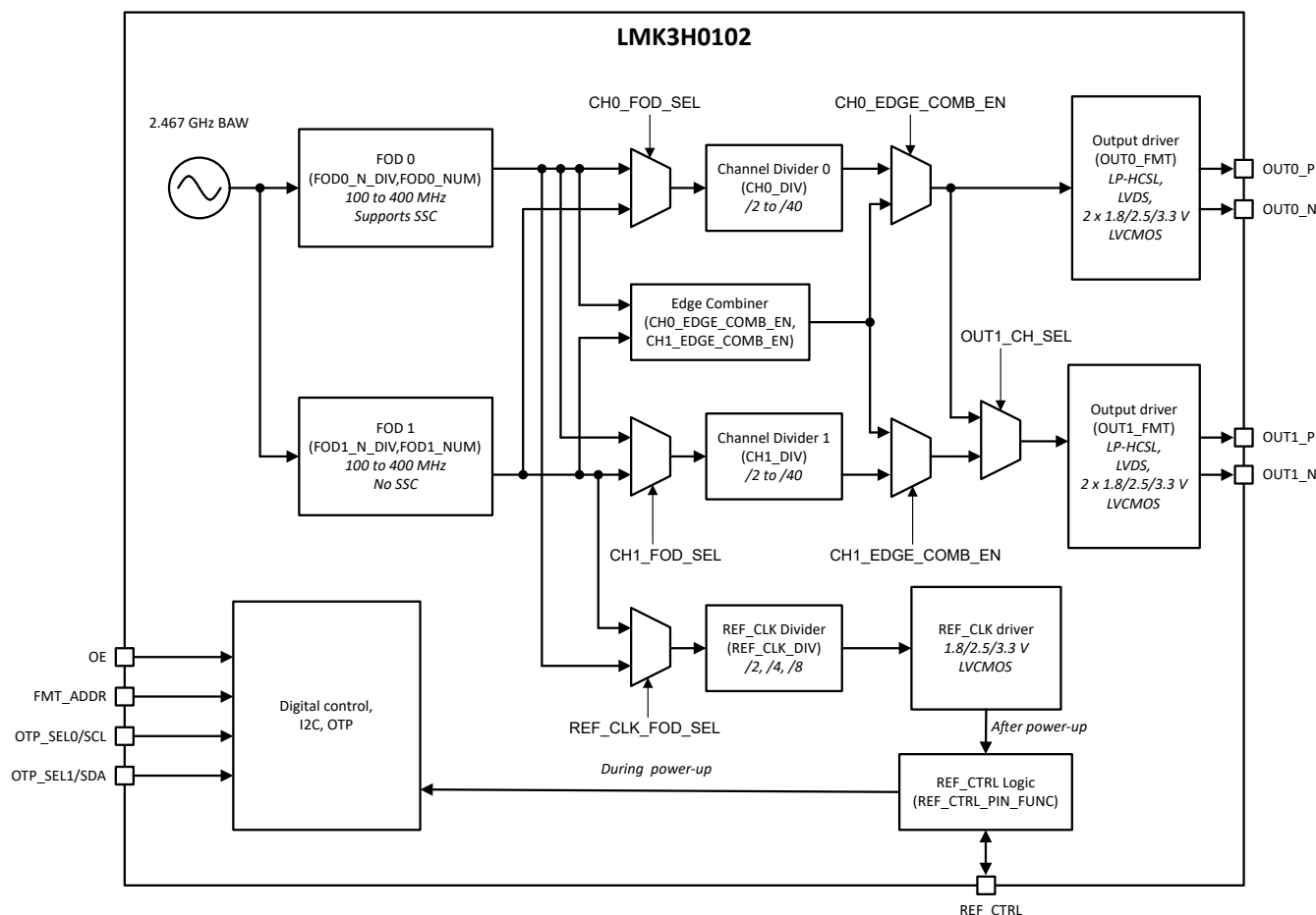
図 7-1. LMK3H0102 の機能ブロック図
