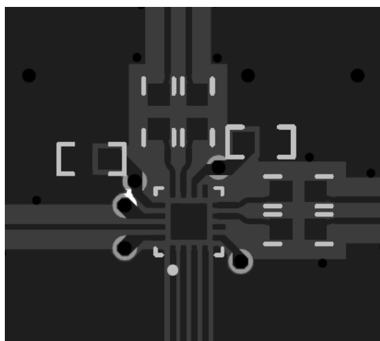
図 9-8. LMK3H0102 の PCB レイアウト例、最上層
