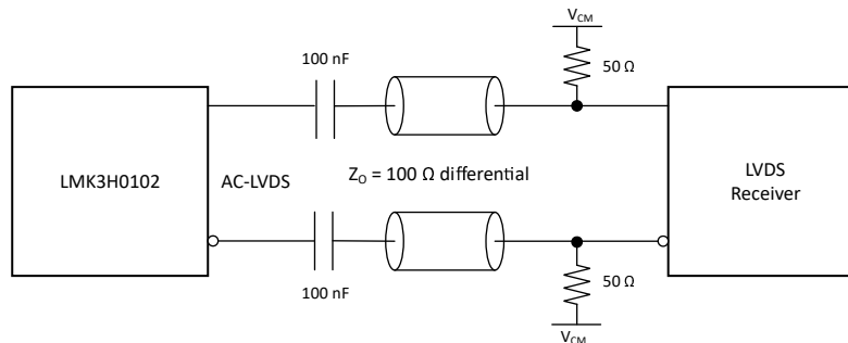
図 7-6. LMK3H0102 の LVCMOS 出力と AC-LVDS レシーバのインターフェイス
