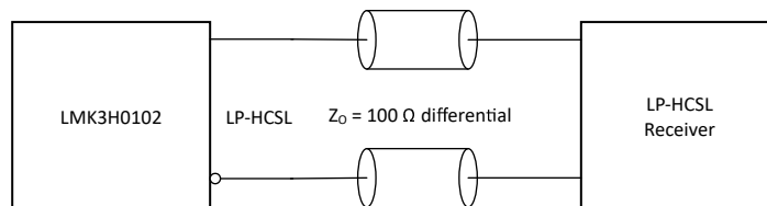
図 7-8. LMK3H0102 の LVC MOS 出力と LP-HCSL レシーバのインターフェイス
