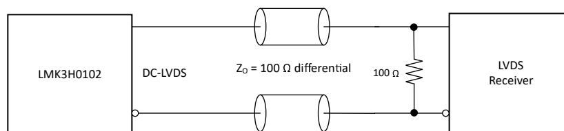
図 7-7. LMK3H0102 の LVC MOS 出力と DC-LVDS レシーバのインターフェイス
