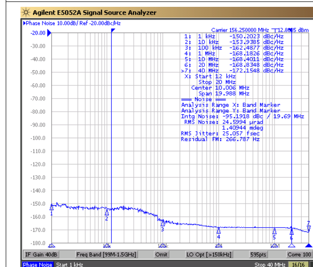
図 6-15. Input Source at 156.25MHz (12kHz - 20MHz)
