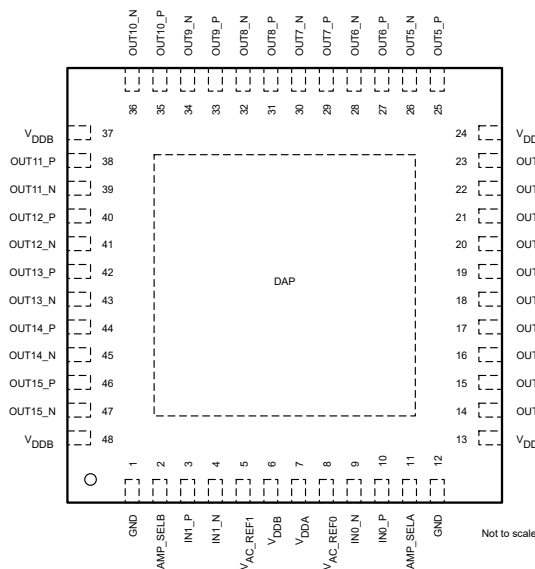
図 5-4. LMK1D2108L: RGZ Package 48-Pin VQFN Top View
