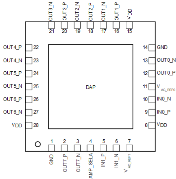
図 5-2. LMK1D2104L: RHD Package 28-Pin VQFN Top View
