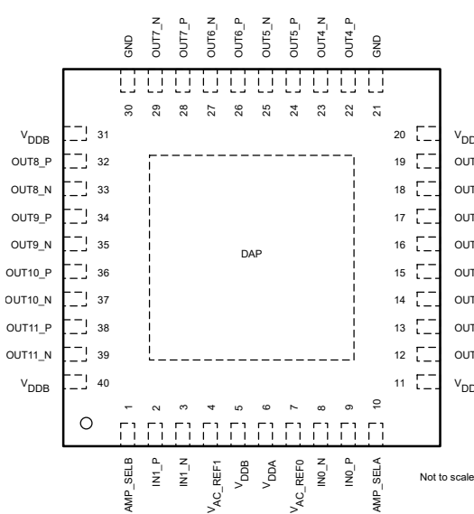
図 5-3. LMK1D2106L: RHA Package 40-Pin VQFN Top View
