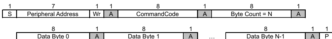
図 9-10. Block Write Protocol
