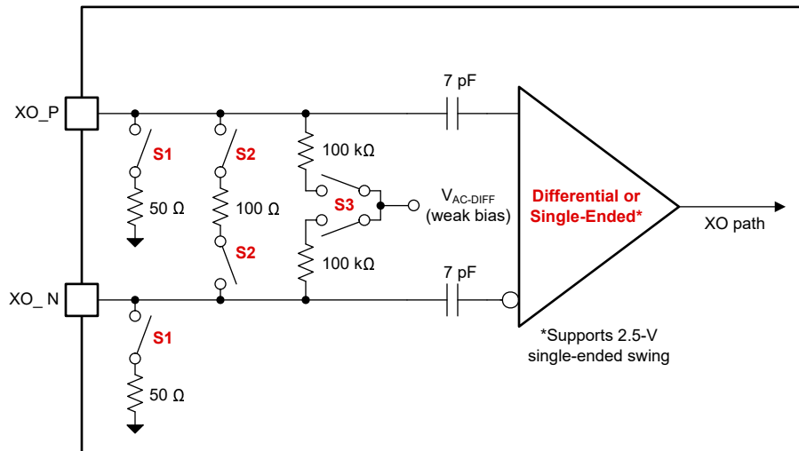
図 7-6. XO Input Buffer
