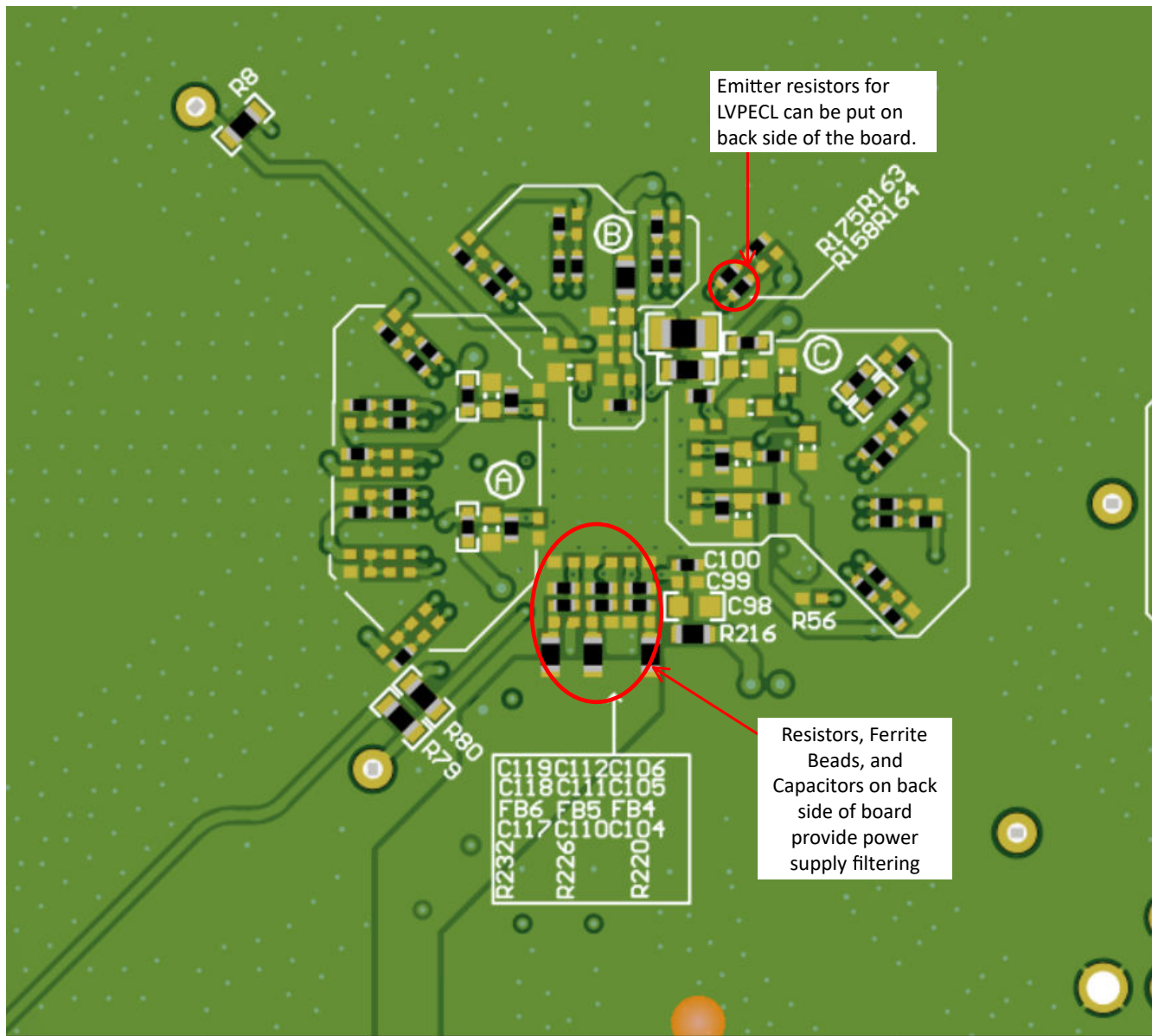
图 9-11. Bottom Layer
