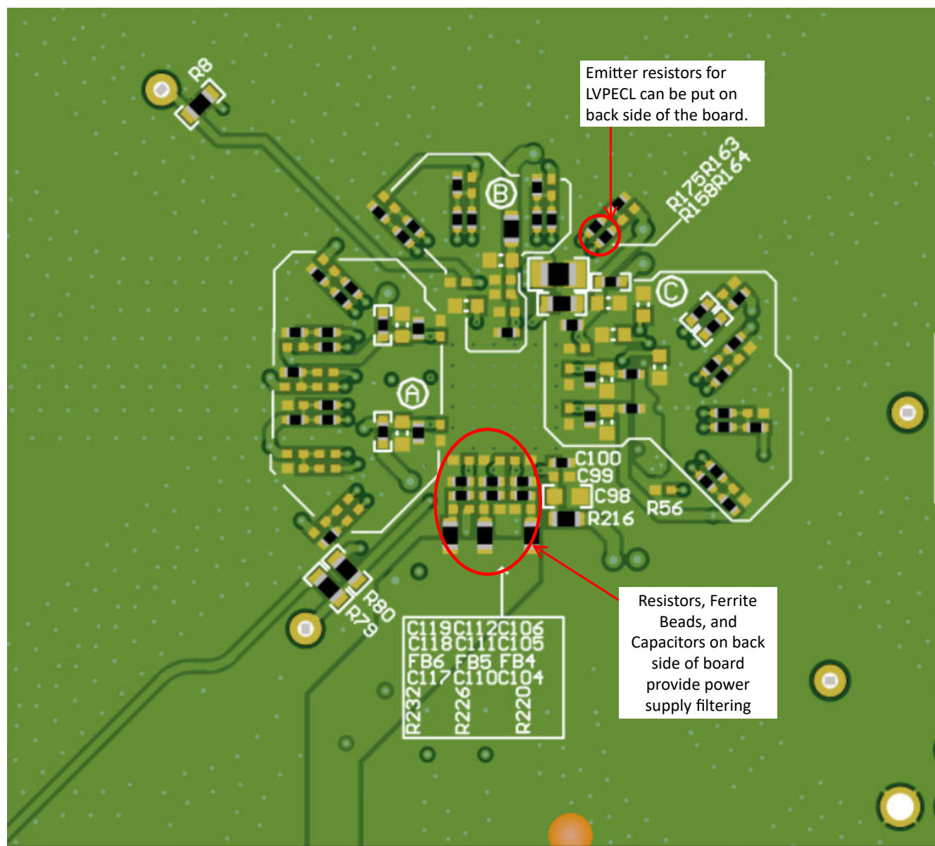
図 9-19. Bottom Layer
