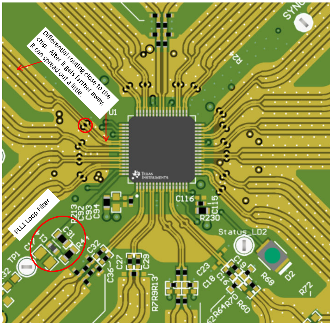
図 9-18. Top Layer
