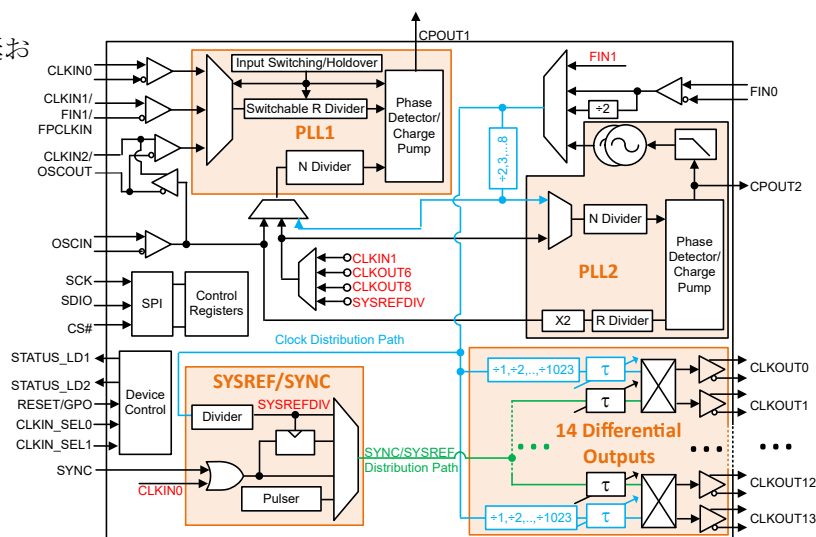
ブロック図
