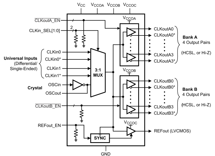
LMK00338 機能ブロック図
