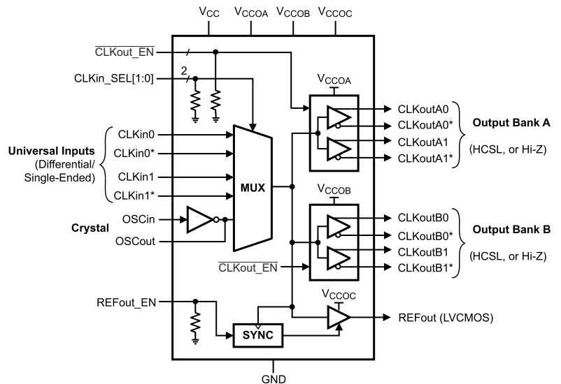
LMK00334 の機能ブロック図
