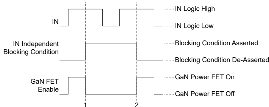
図 7-3. IN 独立ブロッキング状態動作
