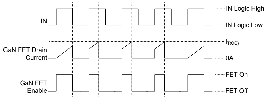
図 7-4. サイクル単位の過電流保護動作
