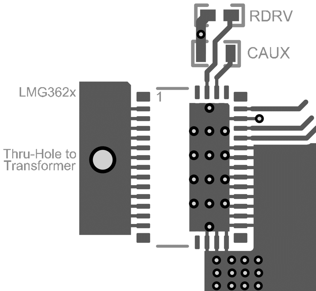
图 8-6. PCB Top Layer (First Layer)
