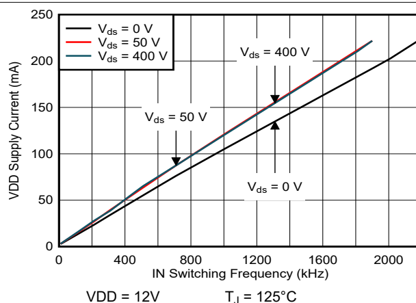
図 5-10. VDD 電源電流と入力スイッチング周波数との関係
