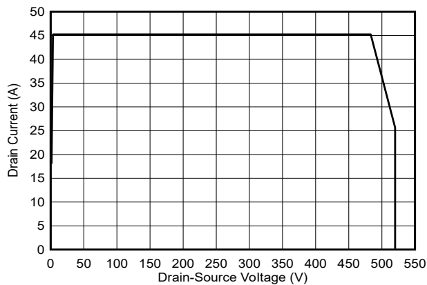
図 5-11. 反復安全動作領域
