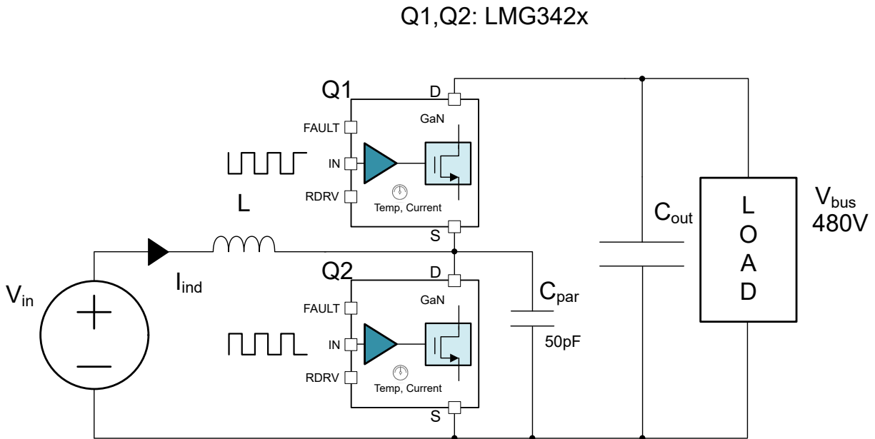
図 6-4. SOA 曲線に使用する回路
