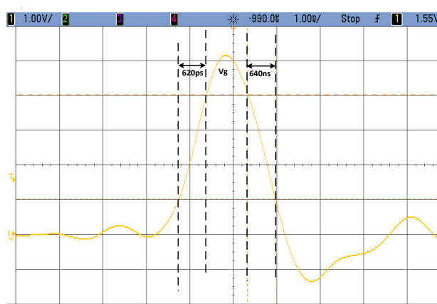
図 7-9. Rise and Fall Time
