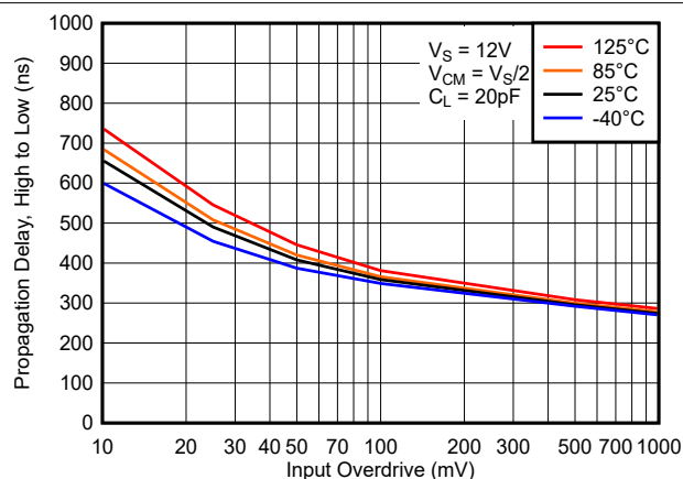
図 5-6. 伝搬遅延、"High" から "Low"、12V
