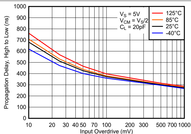
図 5-5. 伝搬遅延、"High" から "Low"、5V
