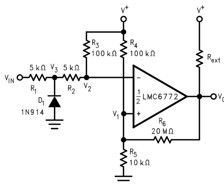
図 6-7. ゼロ交差検出器
