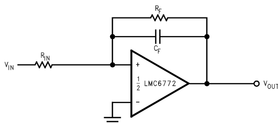
図 6-3. 入力容量の影響の相殺
