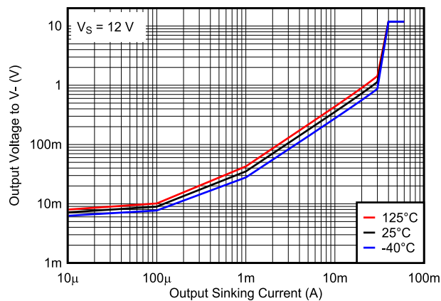
図 5-4. 出力電圧と出力シンク電流の関係、12V
