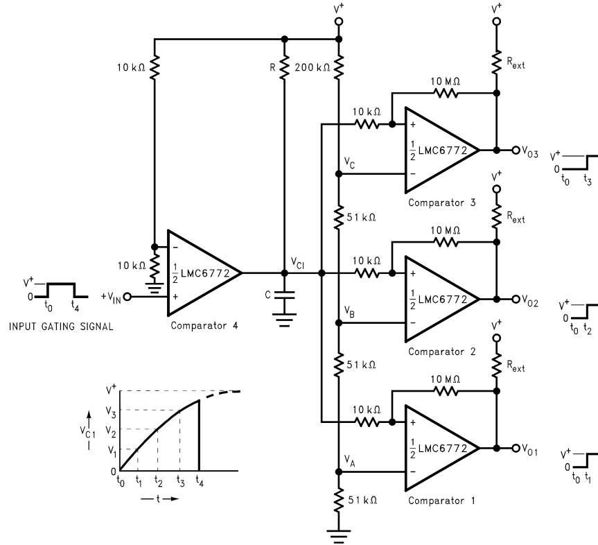
図 6-9. 時間遅延ジェネレータ
