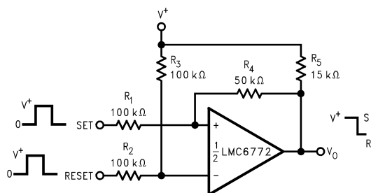
図 6-6. 双安定マルチバイブレータ
