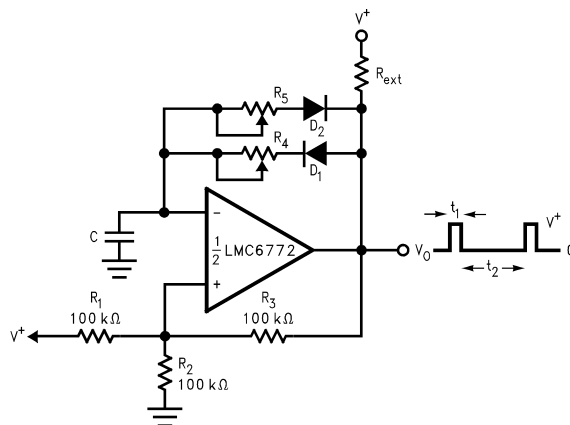
図 6-8. 方形波ジェネレータ
