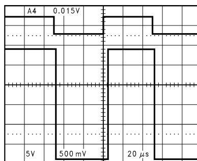
図 6-2. 2.7V の低電源電圧でも、電源電圧を超える入力信号は出力で位相反転なし
