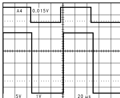
図 6-1. 位相反転なしで、入力信号が LMC6772 の電源電圧を超過
