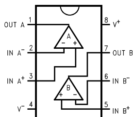
8 ピン PDIP/SOP/VSSOP — 上面図
