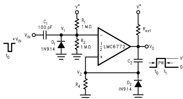
図 6-5. ワンショット マルチバイブレータ
