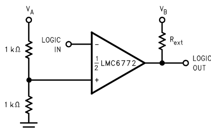
図 6-4. ユニバーサル ロジック レベル シフタ
