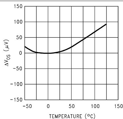
図 5-2. Offset Voltage
