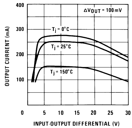
図 5-2. ピーク出力電流
