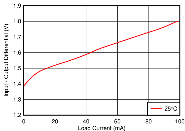
図 7-4. LM78Lxx ドロップアウト
