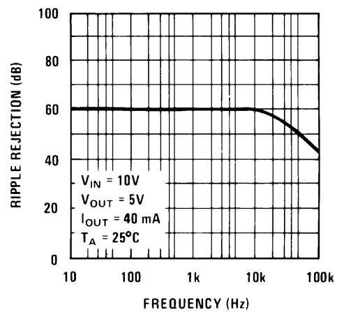
図 5-4. リプル除去
