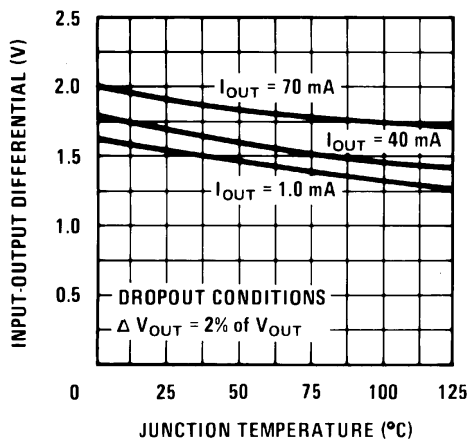
図 5-3. ドロップアウト電圧
