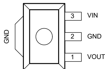
図 4-2. PK パッケージ 3 ピン SOT-89 上面図
