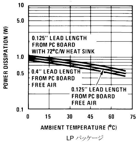
図 5-1. 最大平均消費電力
