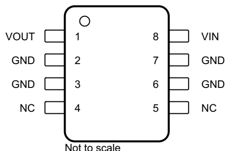
図 4-1. D パッケージ 8 ピン SOIC 上面図
