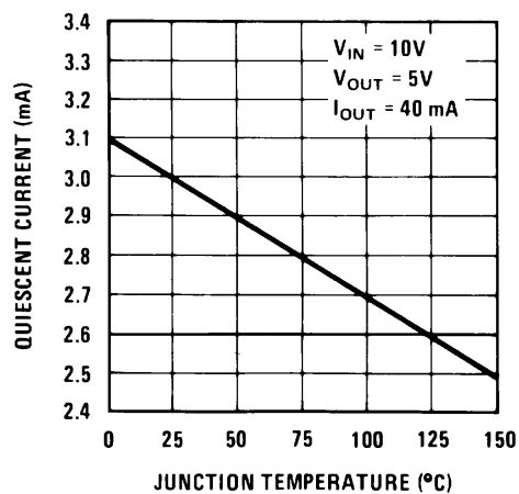
図 5-7. 静止電流
