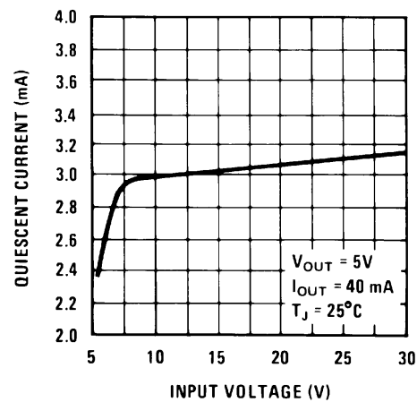
図 5-6. 静止電流
