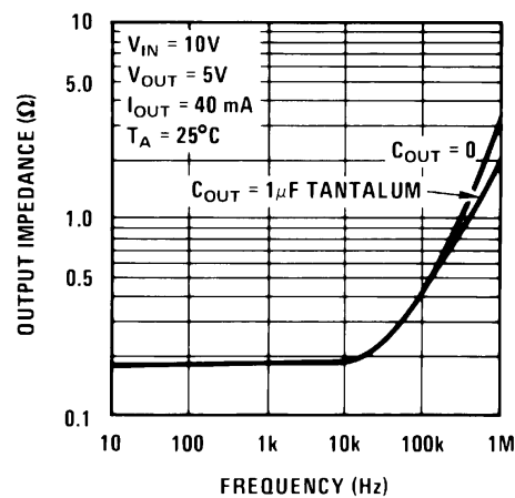
図 5-5. 出力インピーダンス
