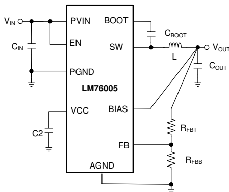
概略回路図
