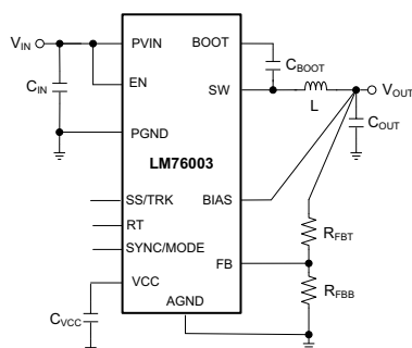
概略回路図
