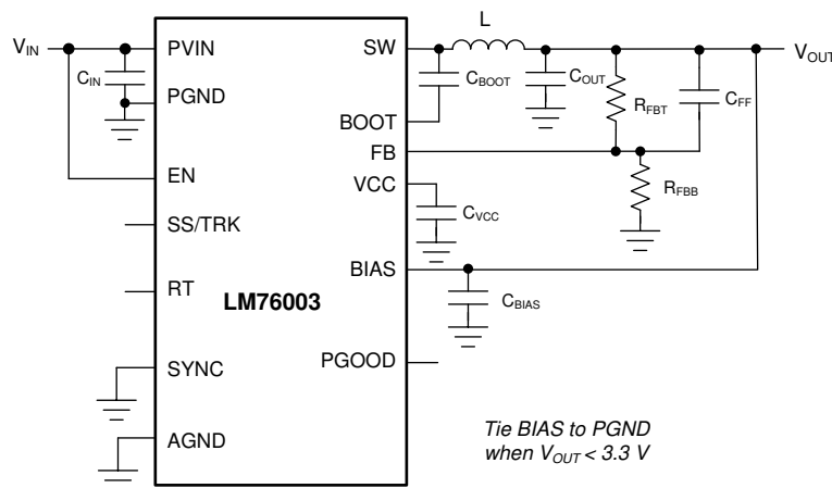
21. LM76002-Q1/LM76003-Q1 Basic Schematic
