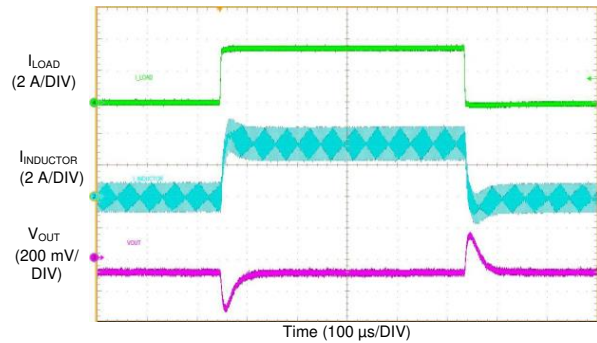
图 74. LM76003 Load Transient
