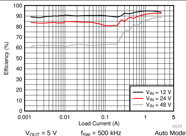
图 35. LM76002 Efficiency
