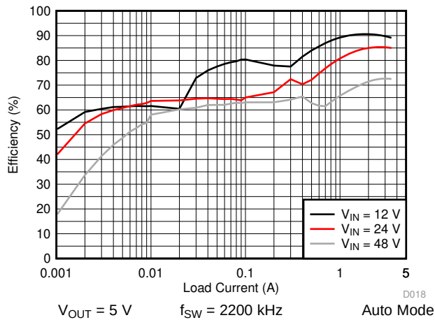
图 29. LM76003 Efficiency
