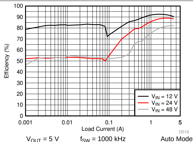
图 27. LM76003 Efficiency
