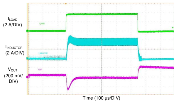
图 77. LM76003 Load Transient
