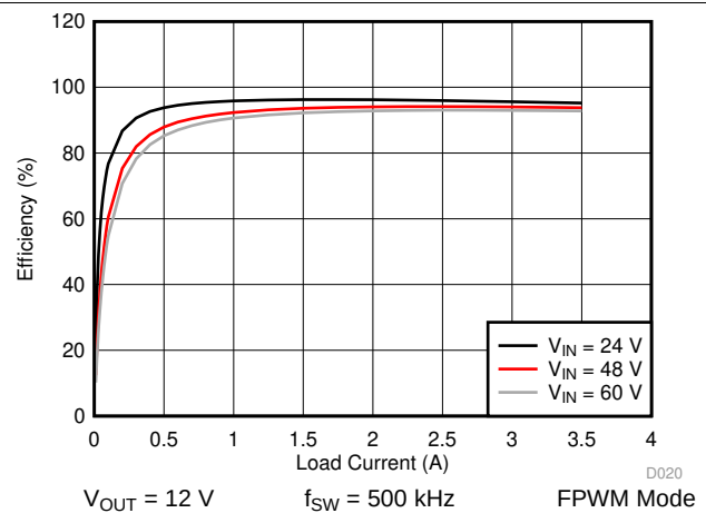
图 32. LM76003 Efficiency
