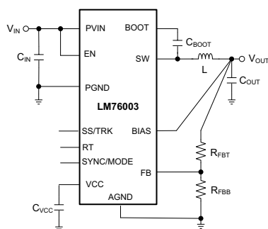
概略回路図
