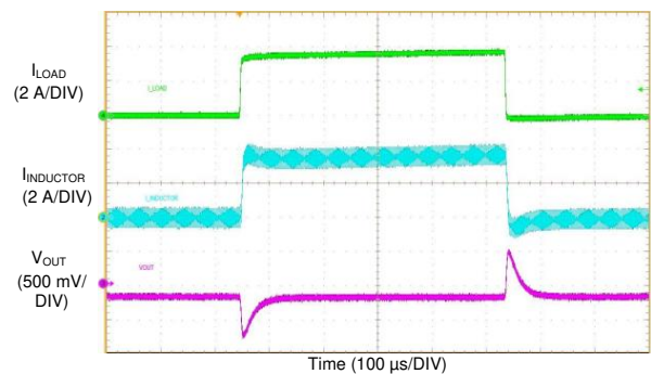
图 80. LM76003 Load Transient
