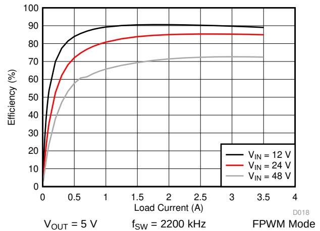
图 30. LM76003 Efficiency
