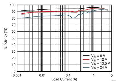
効率と出力電流との関係 ( V_{OUT}=5V 、 f_{SW}=400kHz 、自動モード)
