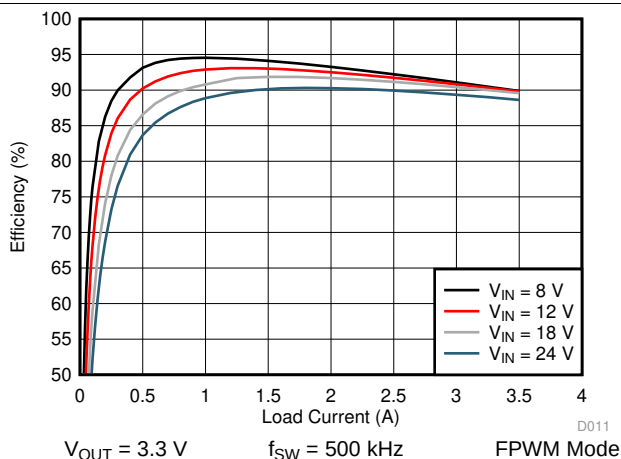
图 24. LM76003 Efficiency
