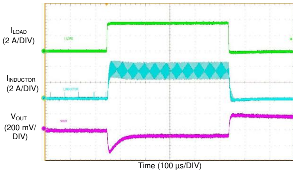
图 73. LM76003 Load Transient
