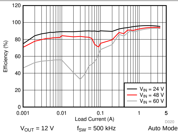
图 31. LM76003 Efficiency
