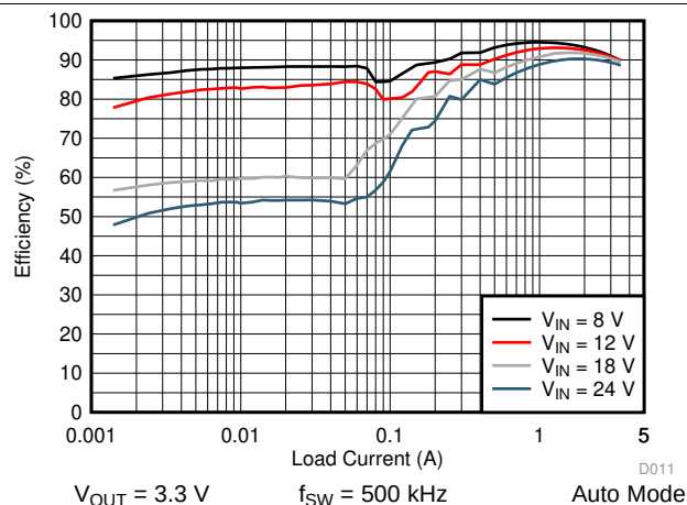
图 23. LM76003 Efficiency
