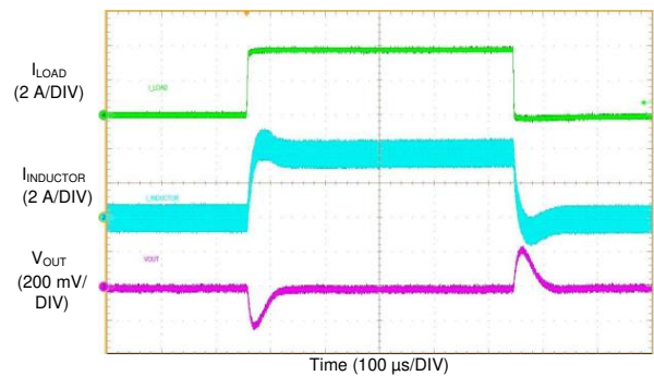
图 78. LM76003 Load Transient
