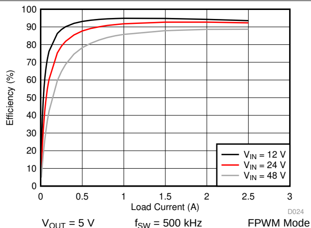
图 36. LM76002 Efficiency
