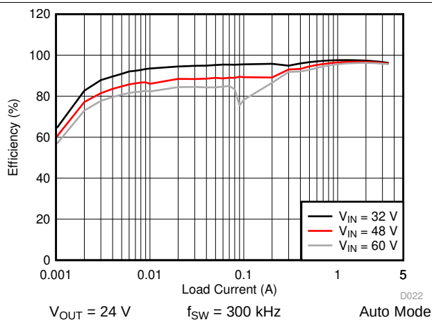
图 33. LM76003 Efficiency
