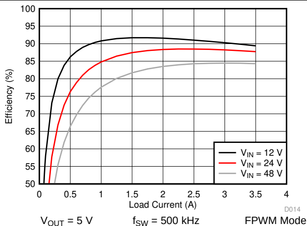
图 26. LM76003 Efficiency
