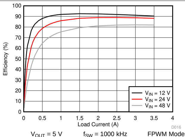
图 28. LM76003 Efficiency
