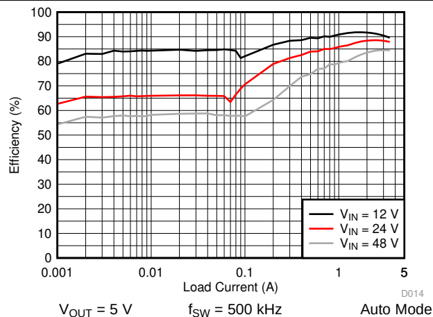
图 25. LM76003 Efficiency
