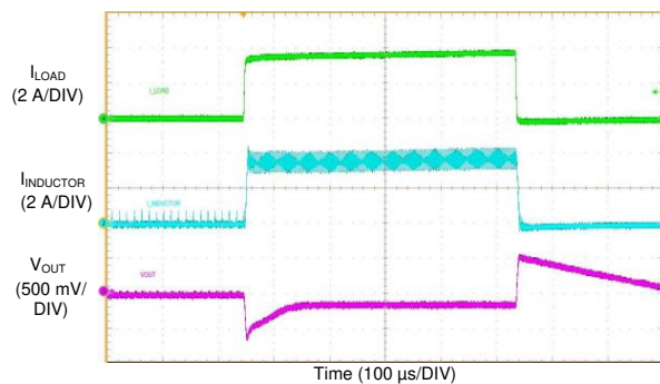
图 79. LM76003 Load Transient
