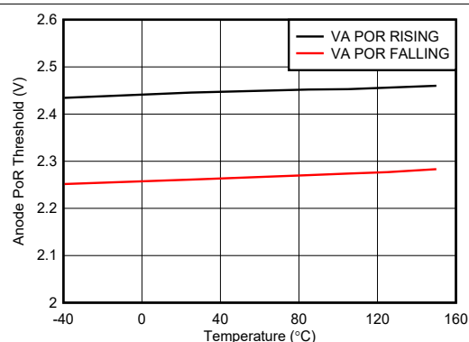
FIG 7-16. VA POR Threshold vs Temperature
