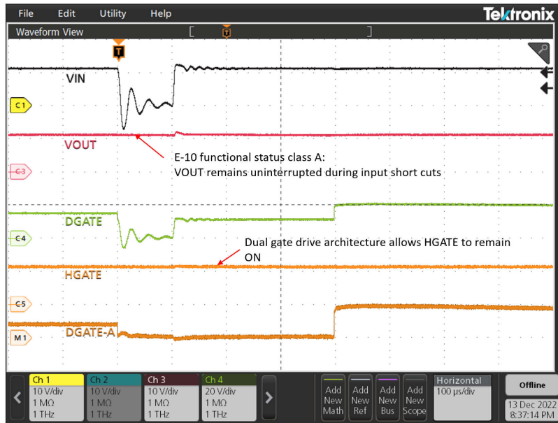
10-5. Input Micro-Short – LV124 E10 TC 2 100 \mu s
