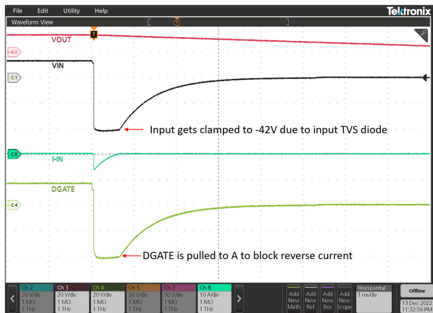
✎ 10-2. ISO 7637-2 Pulse 1
