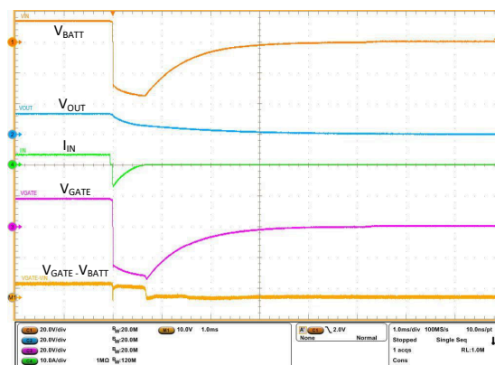
TVS 不要の ISO7637-2 パルス 1 性能
