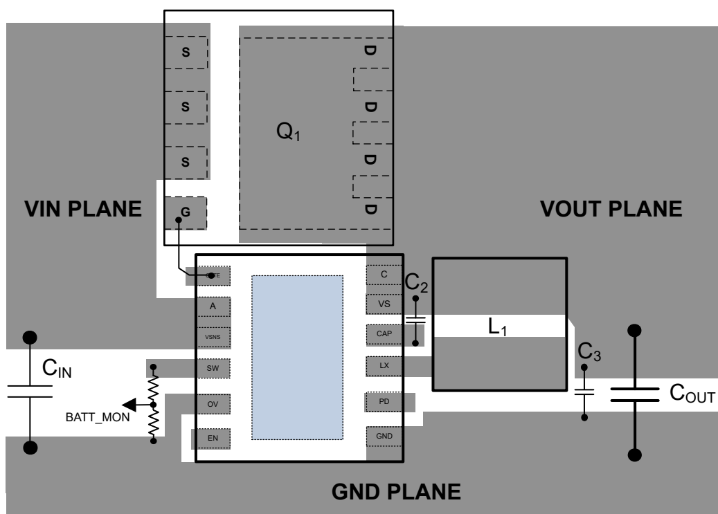
11-1. LM74721-Q1 Layout Example
