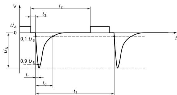
9-4. ISO 7637-2 Pulse 1
