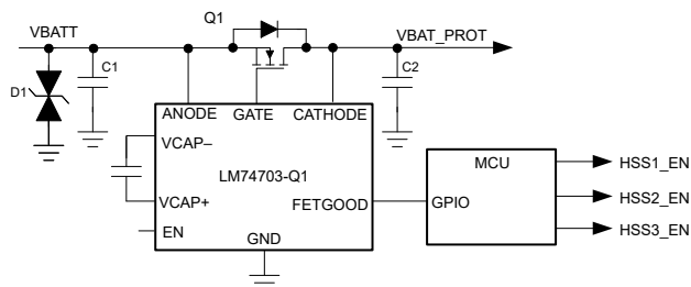
LM74703-Q1 の代表的なアプリケーション回路
