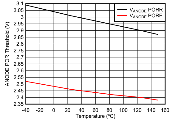
図 6-16. ANODE POR Threshold vs Temperature
