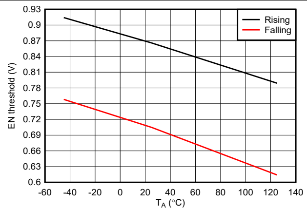
図 5-8. Enable Threshold vs Temperature
