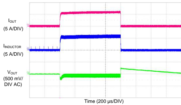
図 69. LM73606 Load Transients
