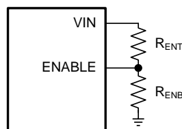
図 14. System UVLO
