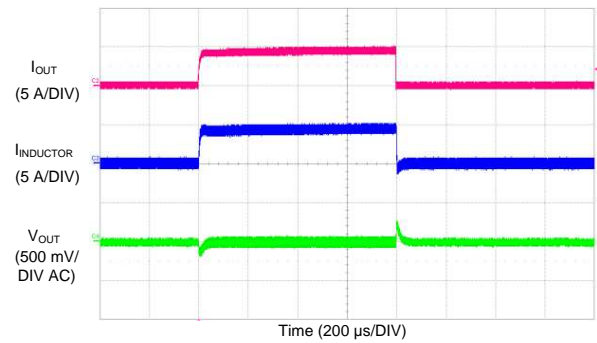
図 70. LM73606 Load Transients
