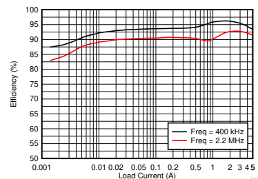
効率と出力電流との関係 ( V_{OUT} = 5\text{V} , V_{IN} = 12\text{V} 、自動モード)
