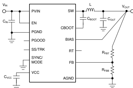
概略回路図
