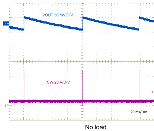
図 7-12. PFM Switching
