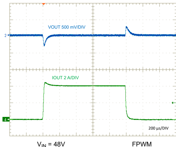
図 7-26. Load Transient, 0A to 4A
