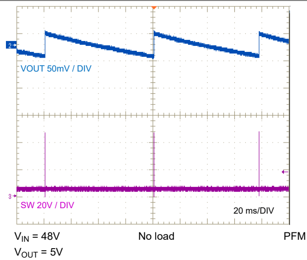
図 7-16. PFM Switching
