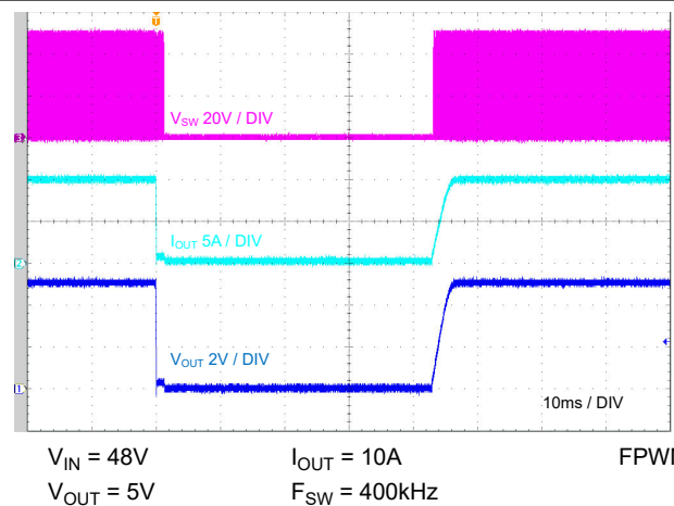
図 5-11. Short-Circuit Recovery
