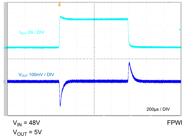
図 5-9. Load Transient, 0A to 5A
